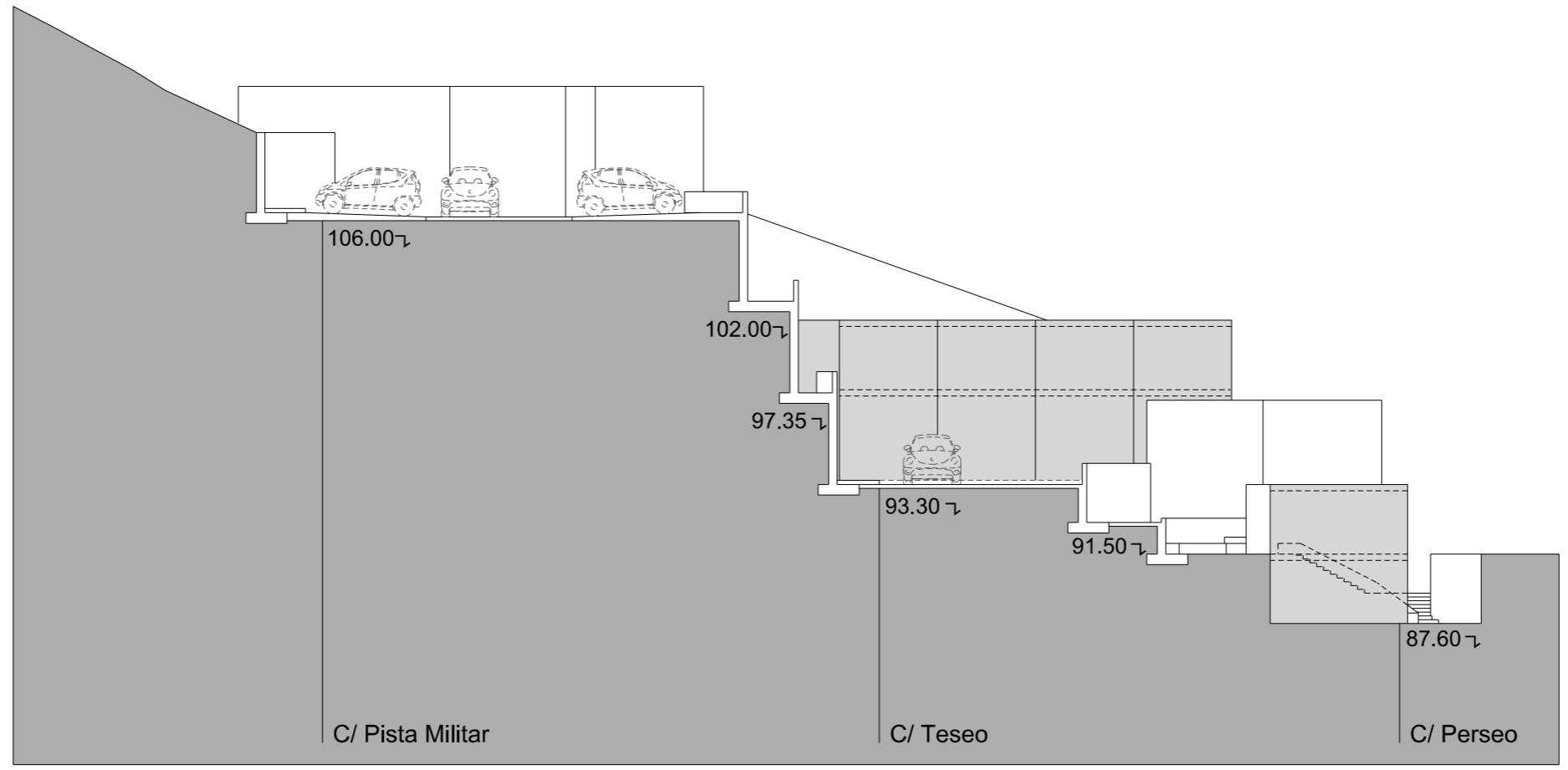
Sección S1
