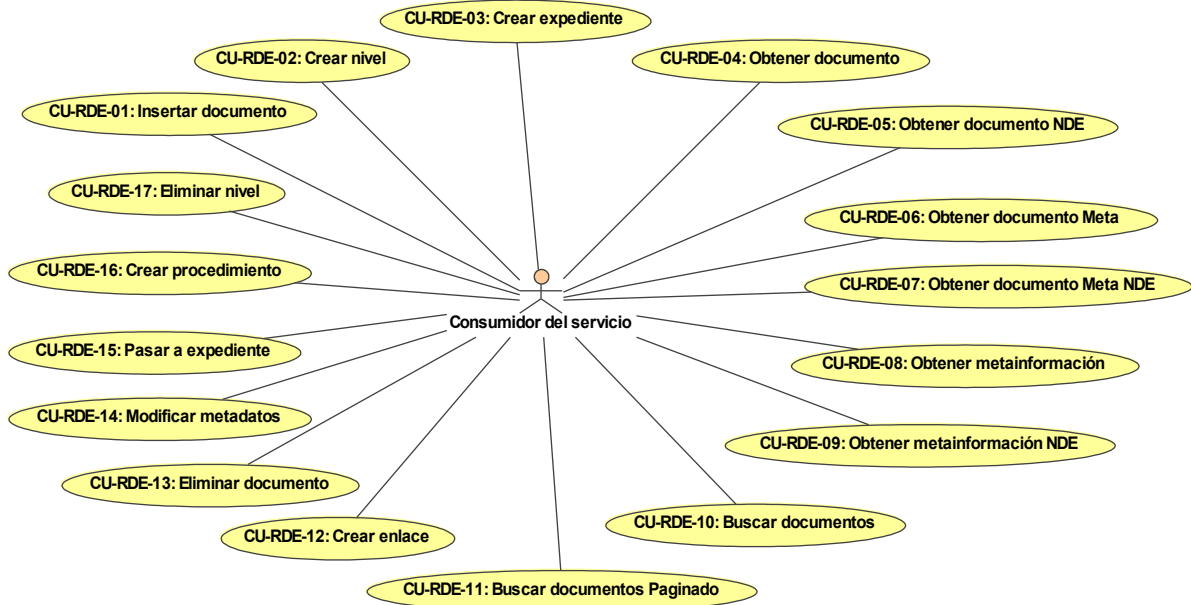
Figura 1: Casos de uso del SGRDE.
