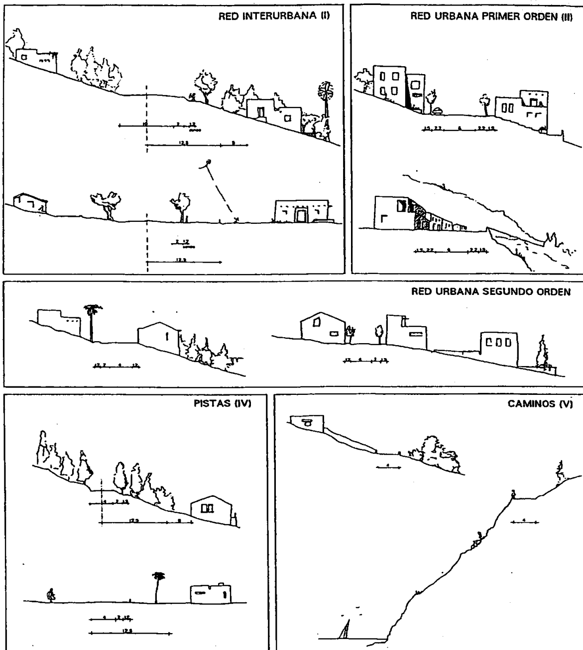
RED VIARIA Y EDIFICACIÓN: DIRECTRICES INDICATIVAS PARA SU DIMENSIONADO (NUEVOS TRAZADOS EN EXTENSIÓN DE NÚCLEOS)
