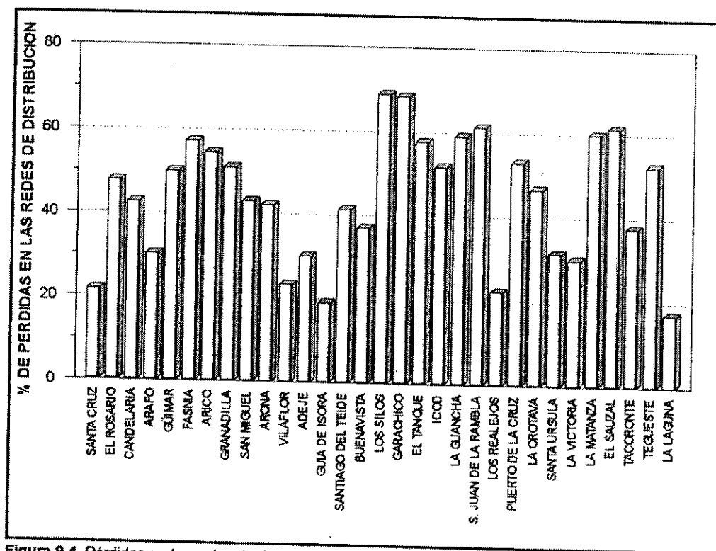
Figura 9.4. Pérdidas en las redes de distribución
